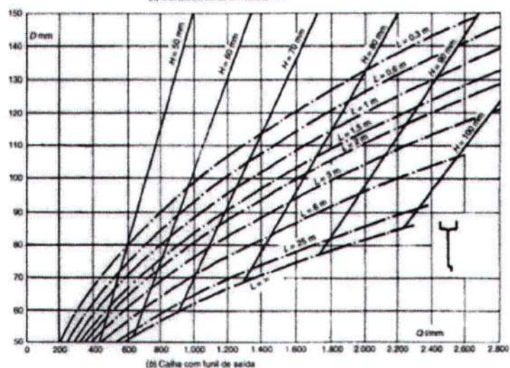
Fig. 3.37 Ábacos para a determinação de diâmetros de condutores verticais.
