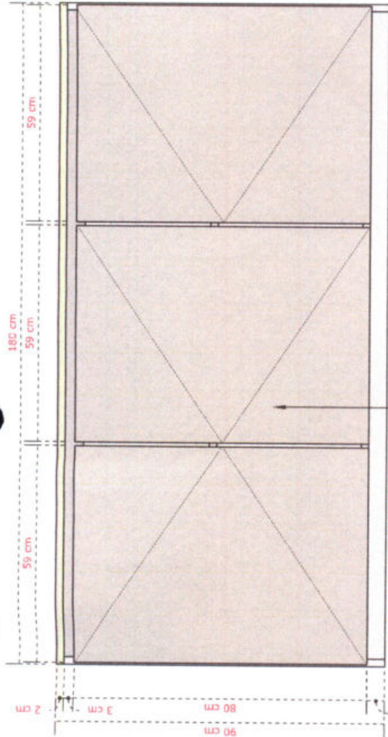
02 - VISTA FRONTAL MB23 ESCALA.....1/10
