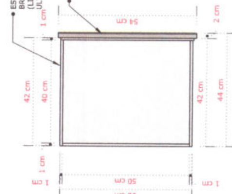
01 - VISTA INTERNA MB27 ESCALA.....1/10
