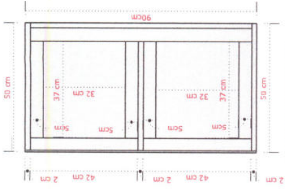
04 - VISTA SUPERIOR MB1 ESCALA.....1/10
