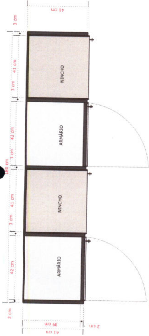
02- PLANTA BAIXA MB24 ESCALA.....1/10
