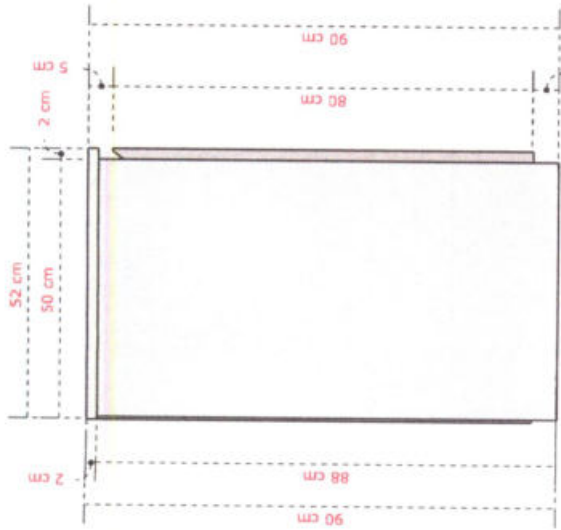
01 - VISTA INTERNA MB23 ESCALA.....1/10
