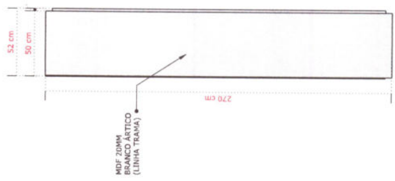
02 - VISTA LATERAL MB14 ESCALA.....1/20
