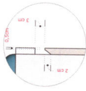
05 - DET. PUXADOR CAVA MB22 ESCALA.....1/10
