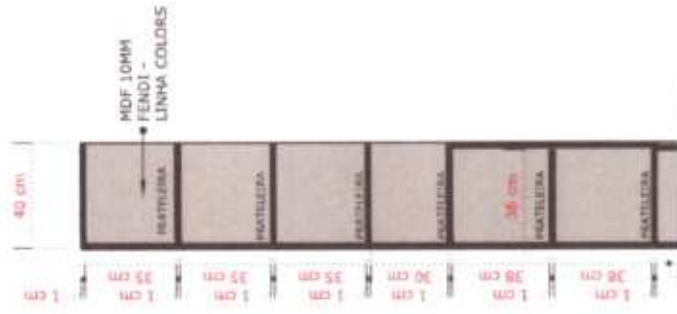
05 - CORTE MB9 ESCALA.....1/20
