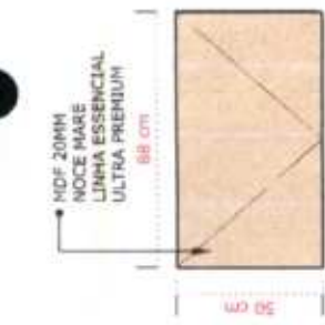
02- VISTA FRONTAL MB28 ESCALA.....1/20
