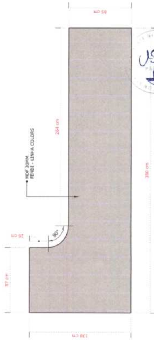
04- VISTA SUPERIOR PEÇA 2 MB10 ESCALA.....1/20
