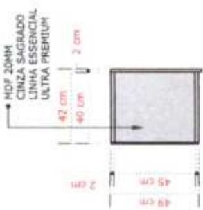
01- VISTA LATERAL MB28 ESCALA.....1/20
