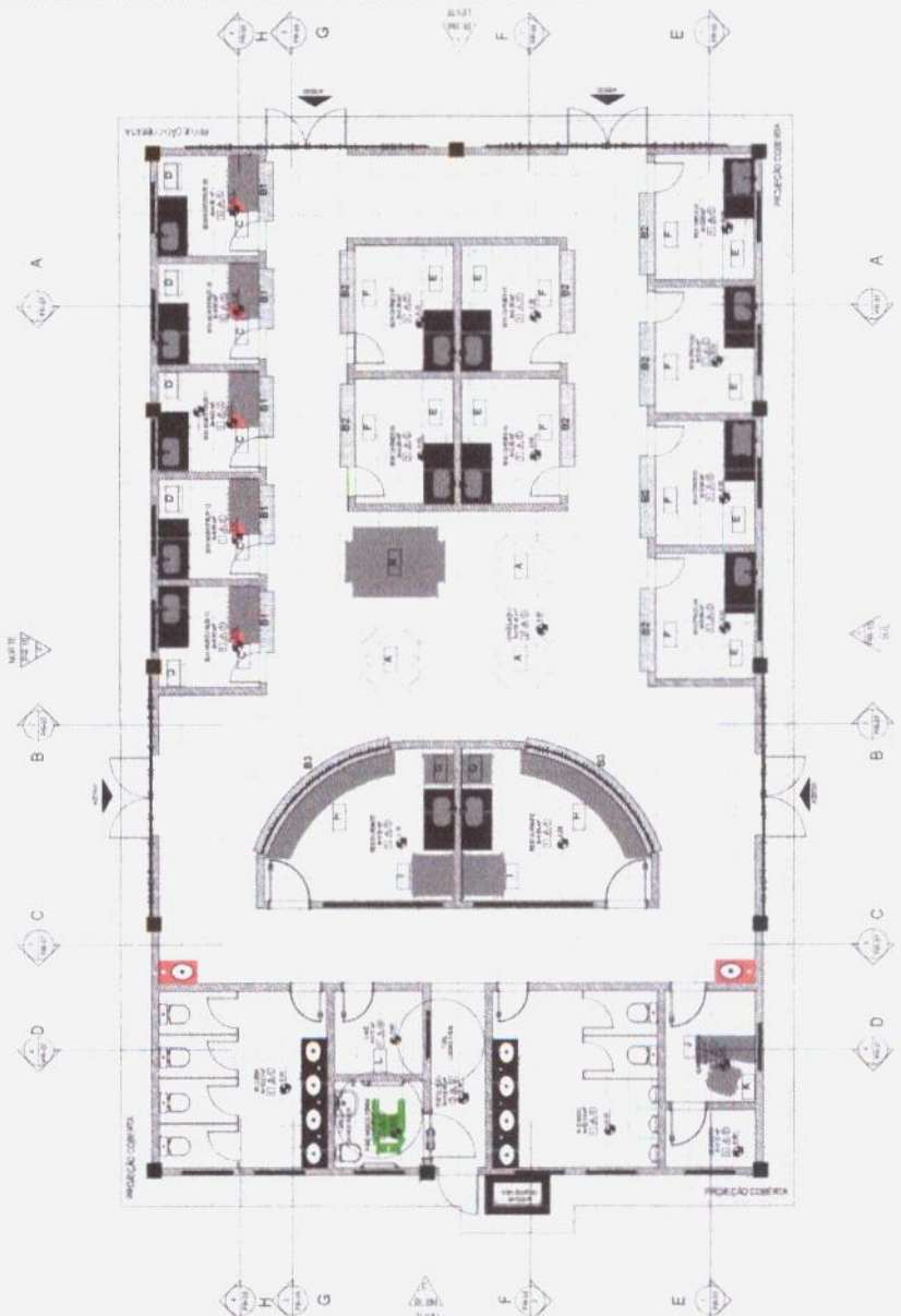
1 PLANTA DE LAYOUT
