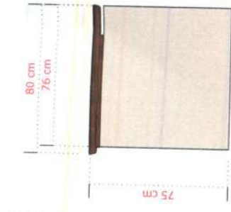
02 - VISTA 1 MB4 ESCALA.....1/20
