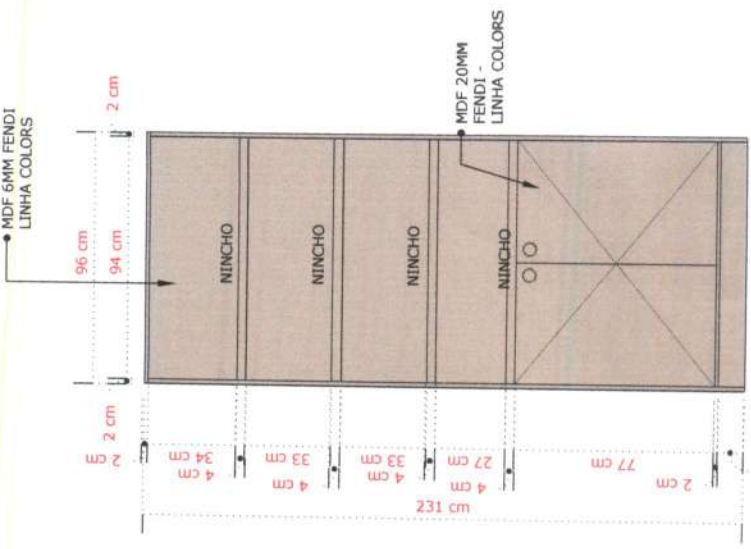
06 - VISTA 2 MB11 ESCALA.....1/20
