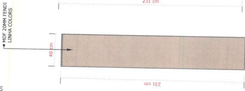
05 - VISTA 1 MB11 ESCALA.....1/20
