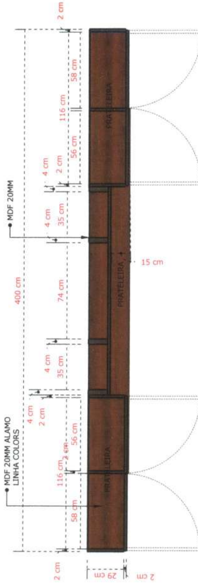
03 - PLANTA MB21 ESCALA.....1/20
