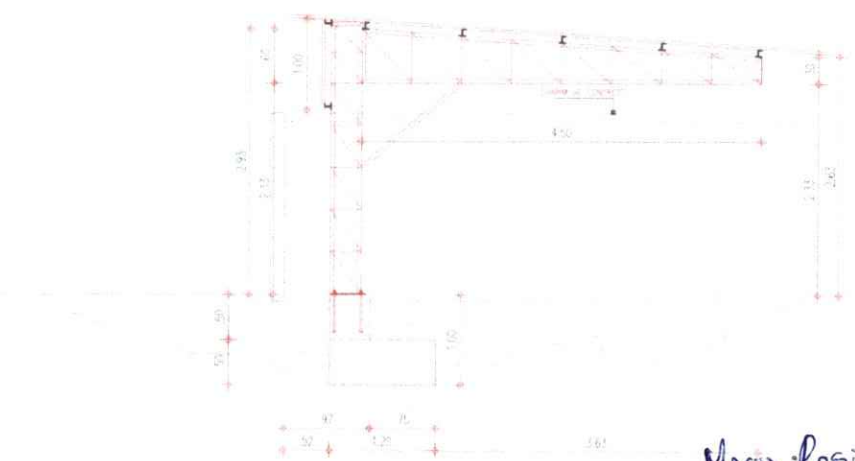
CORTE LATERAL COBERT. 01
