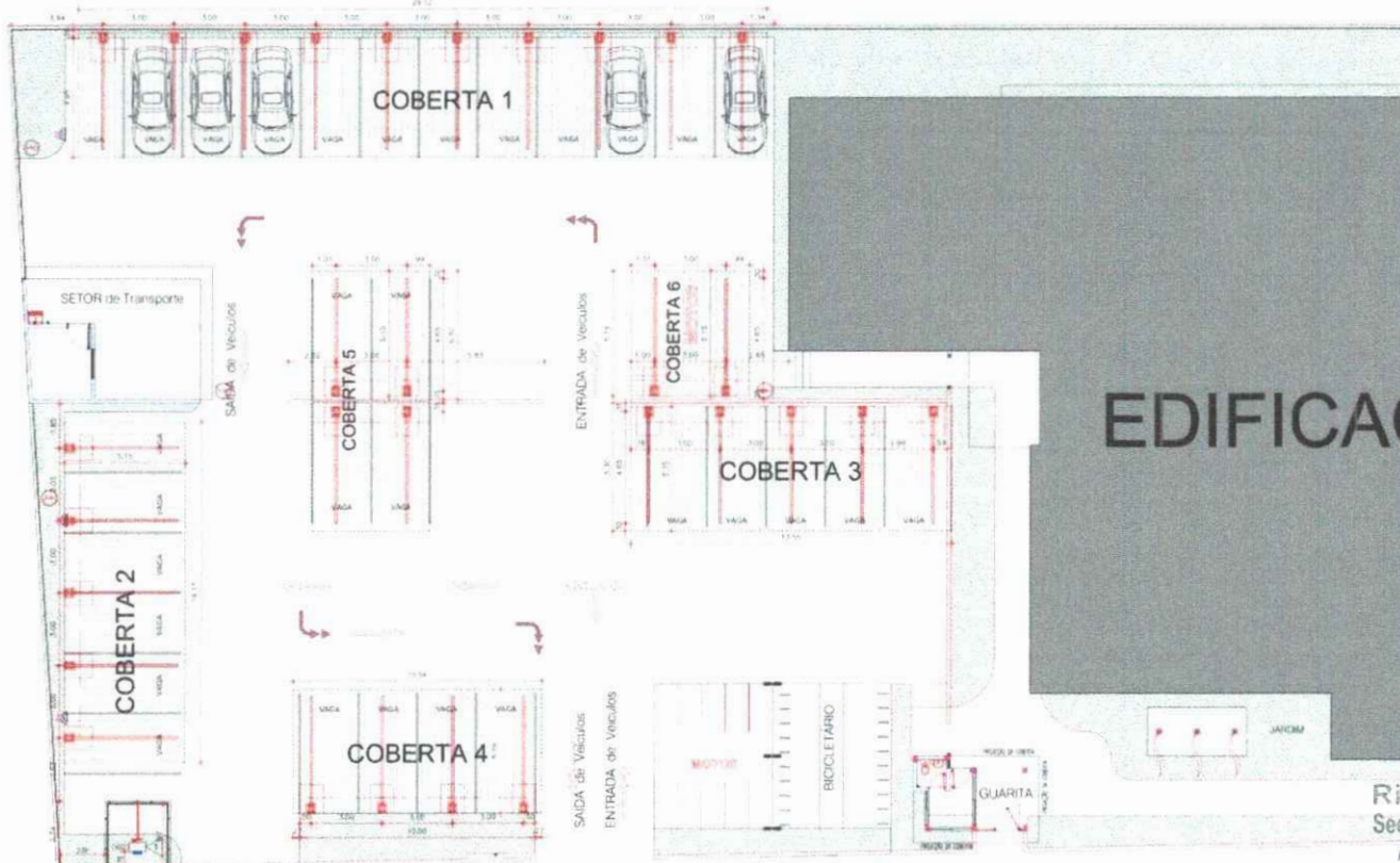
01 PLANTA DE LOCAÇÃO (ESCALA 1:100)
