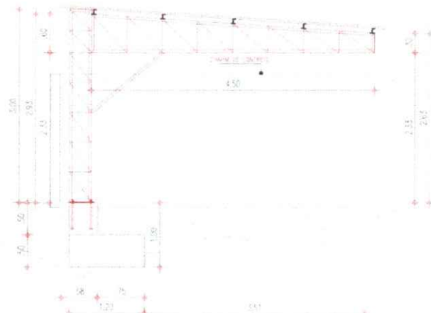
CORTE LATERAL COBERT. 04
