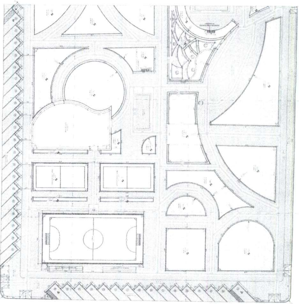
1 - PLANTA TÉCNICA SETOR 1
