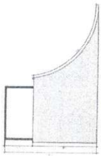
2 CORTES OBSTÁCULO A - PISTA DE SKATE
